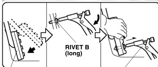
BRAKE PEDAL
